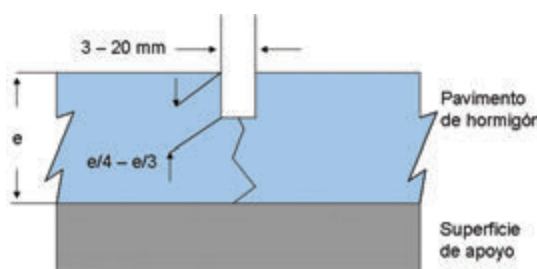
Junta de contracción
